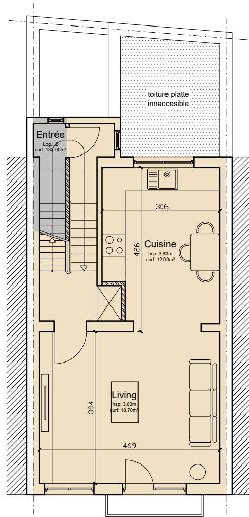
ETAGE 1
