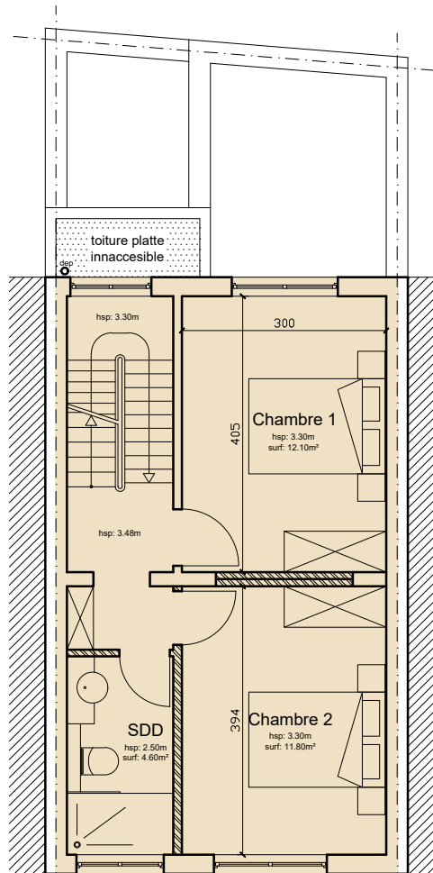
ETAGE 2
